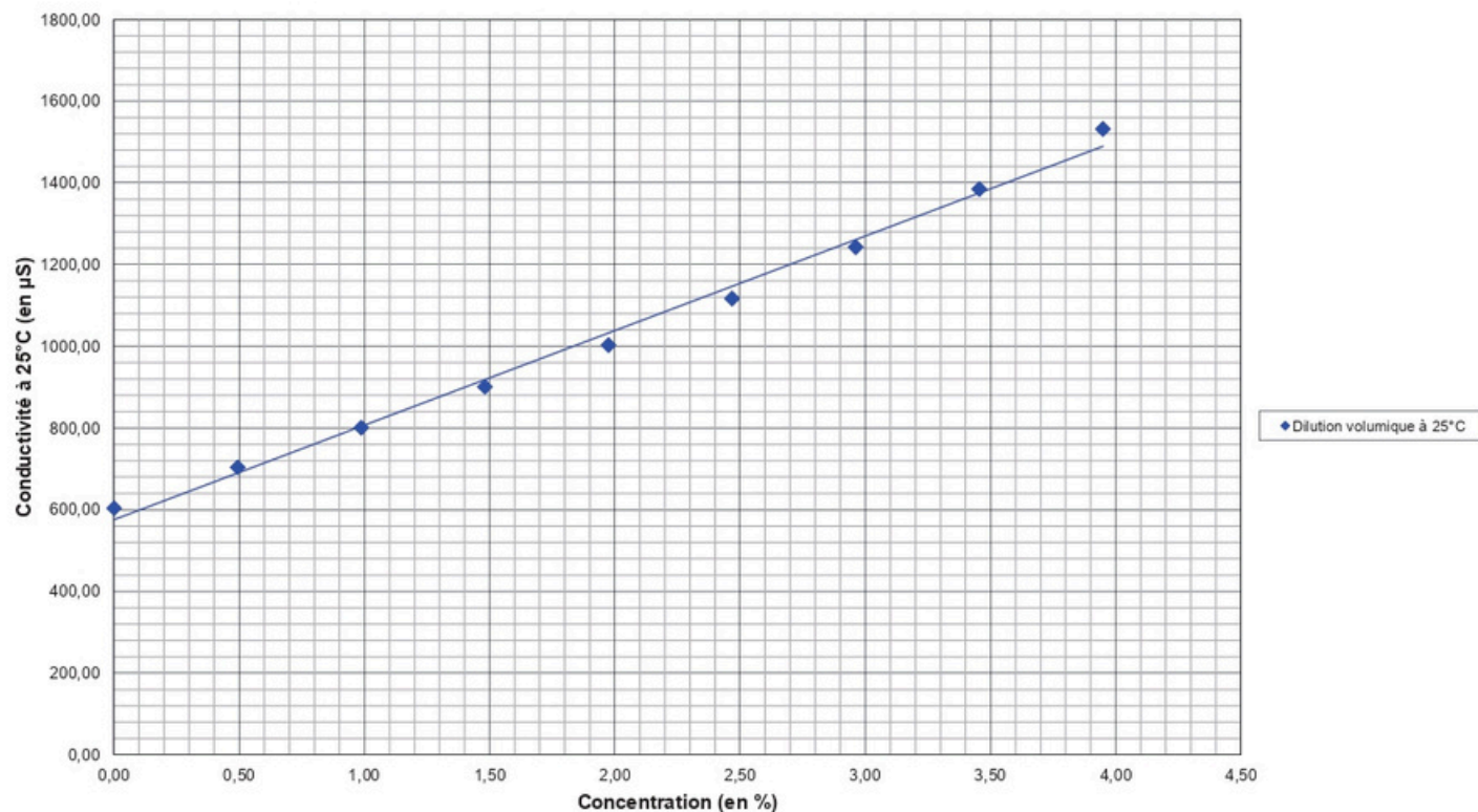
Courbe de conductivité à 25°C du PRO BACT DDM+ ELEMAL'AL Courbe réalisée avec une eau de dureté = 18°f avec le conductimètre WTW Cond 3110
